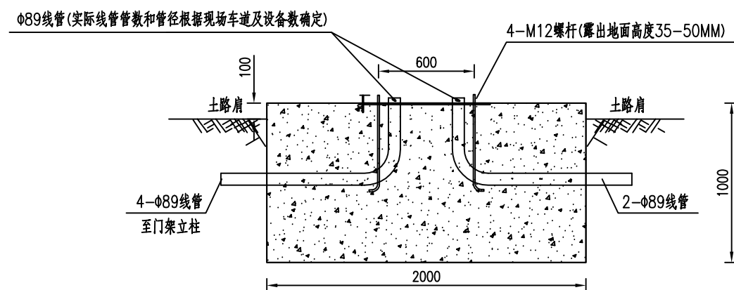
基础立面图
