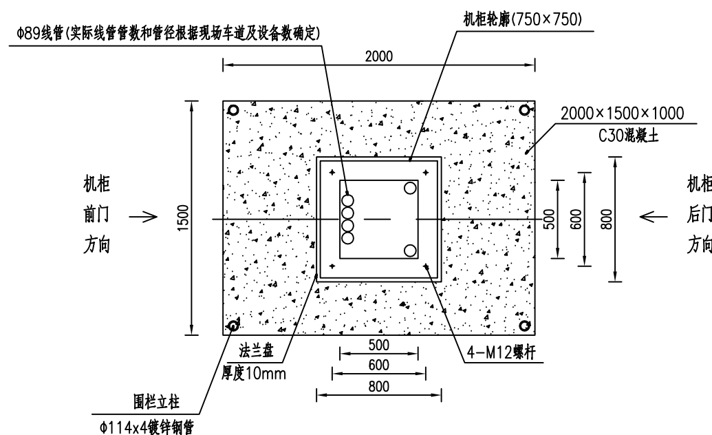
基础平面图
