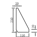
底法兰角筋 \delta=15
