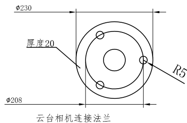
云台相机连接法兰
