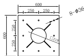
底法兰 \delta=20
